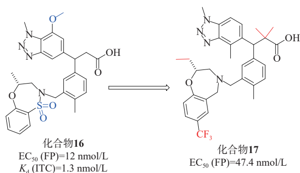
图 7 化合物 16 、 17 的结构式
