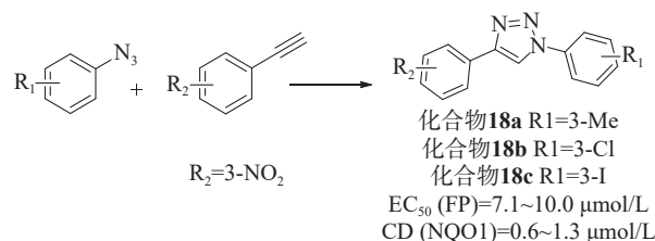
图 8 化合物 18a 到化合物 18c 的设计思路
