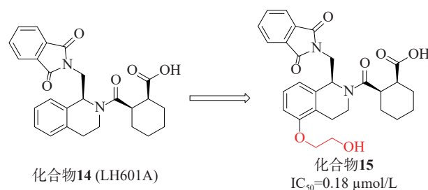
图6 化合物14、15的结构式
