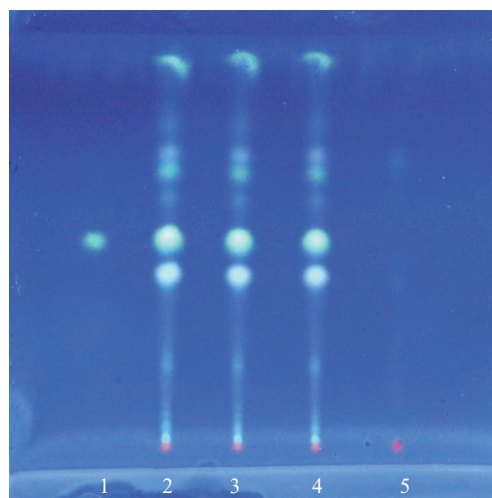
图 1 密蒙花的薄层色谱图
