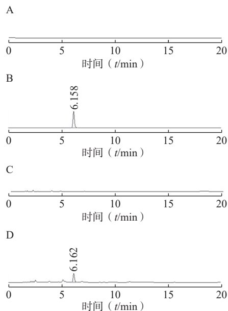
图1 四草克银凝胶液相色谱图
