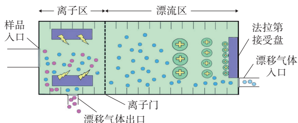
图 1 气相色谱-离子迁移谱联用技术分离示意图
