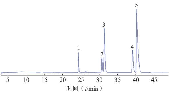
图 2 混合对照品 HPLC 图谱
