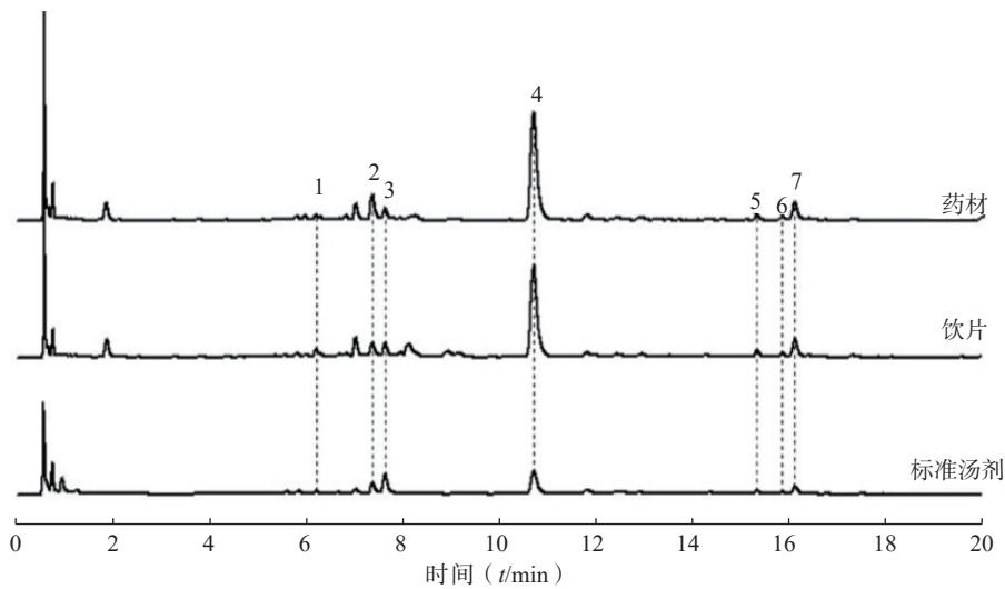
图 4 穿心莲药材-饮片-标准汤剂的特征图谱对比图
