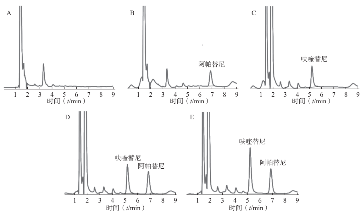
图 1 血浆样品的 HPLC 色谱
