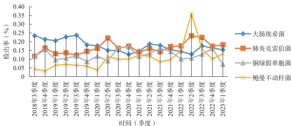
图1 2018年第3季度至2023年第1季度G - 菌构成比各季度检出折线图
