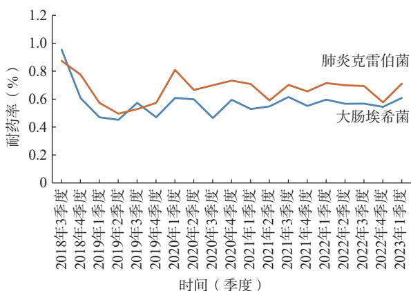
图 3 大肠杆菌和肺炎克雷伯菌头孢唑林耐药率折线图
