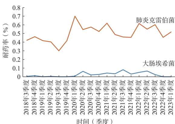
图 2 大肠杆菌和肺炎克雷伯菌亚胺培南耐药率折线图
