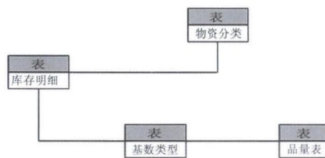
图1 相关数据字典的关联方式设计
